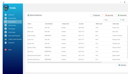
Gambar 8. Menu Kelahiran
