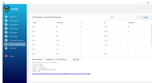
Gambar 13. Menu Prediksi
