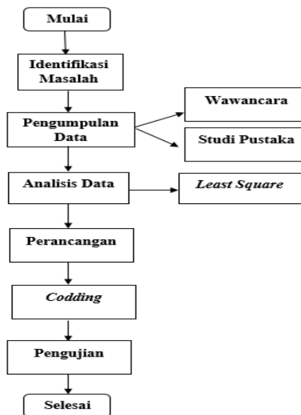
Gambar 2. Tahapan Penelitian
