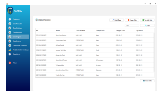
Gambar 10. Menu Imigrasi
