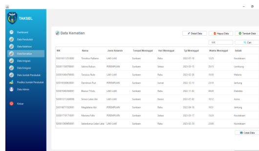
Gambar 9. Menu Kematian
