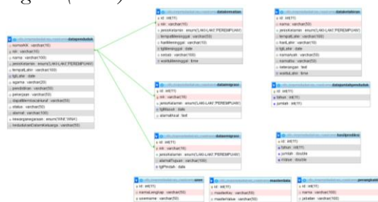
Gambar 4. ERD TAKSEL
